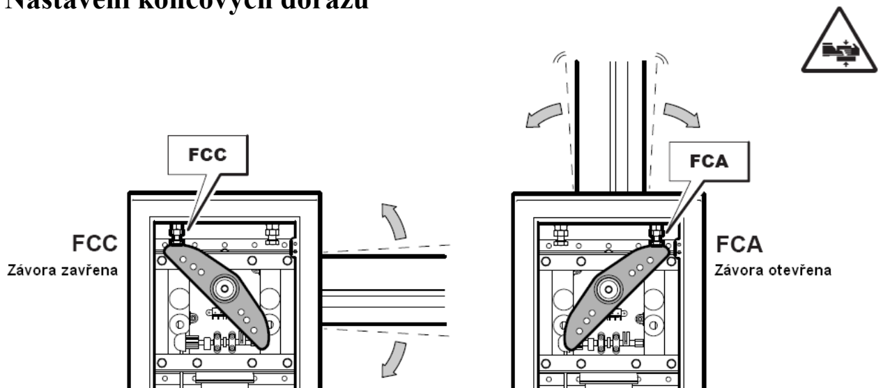
Montáž břevna a nastavení koncových dorazů na levé závoře
